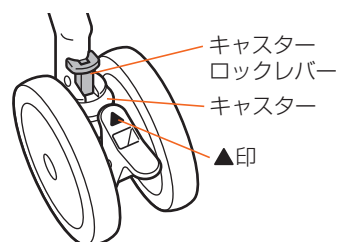
図B 押す人側のストッパーの▲印がキャスターロックレバーと向きあい、キャスターが確実にロックされていることを確認
