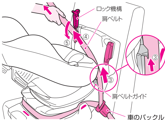
ロック機構の開閉のしかた
