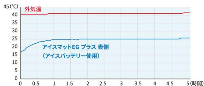
●「アイスバッテリー」性能テスト・検証結果
