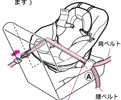
ロッキングクリップ 取り付け位置
